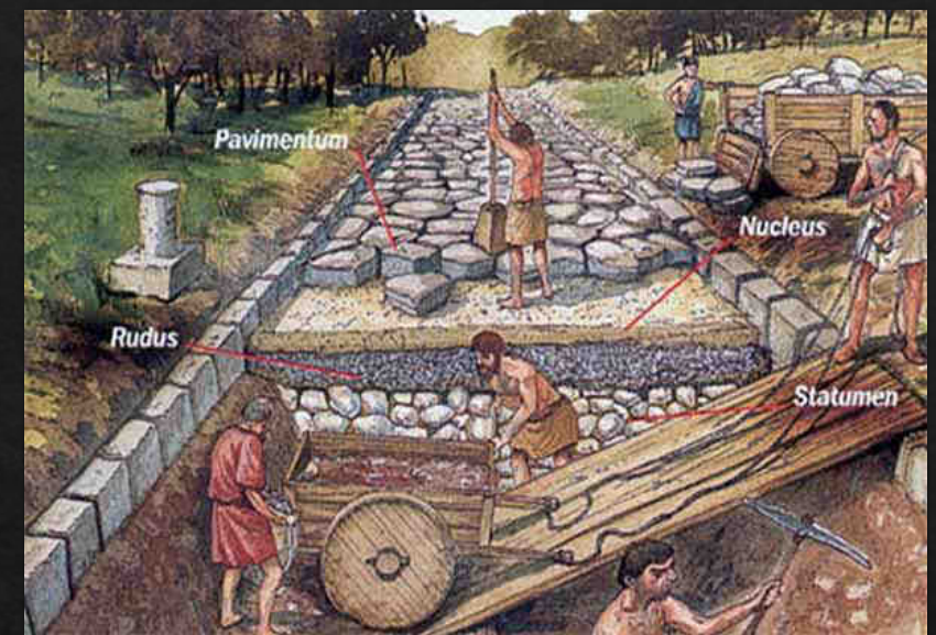
Modalità di costruzione di una strada lastricata
